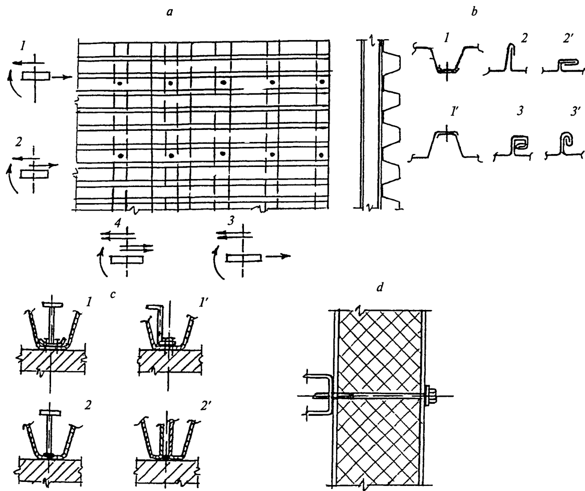
а - фрагмент конструкции покрытия со стальным профилированным настилом и схема действия сил на опорах (1 - соединения в среднем участке; 2 и 3 - соединения соответственно по продольным и поперечным полкам; 4 - соединения в месте пресечения продольных и поперечных полок); б - схема соединений по продольным полкам (1 и 1' - при расположении полок внахлест в нижнем и верхнем положениях соответственно для утепленных и холодных покрытий; 2 и 2' - простой стоячий и лежачий фальцы; 3 и 3' - варианты двойного фальца); в - сдвигустойчивые элементы (1 и 1' - на высокопрочных дюбелях; 2 - на контактной сварке; 2' - на дуговой сварке); д - фрагмент трехслойной стеновой панели на самосверлящем винте
