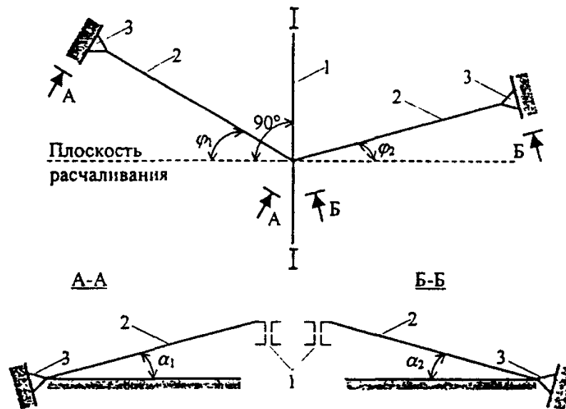
Рисунок А.2 - Схема раскрепления ферм расчалками
